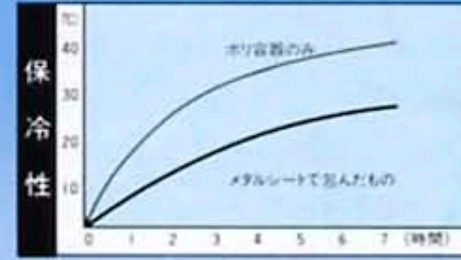
注)ポリ容器(500cc)に冷水(2℃)を入れ、40℃の室温に置き経過時間による温度変化を測定した。
