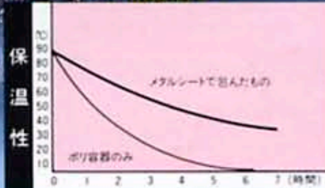
注)ポリ容器(500cc)に温湯(88℃)を入れ0-5℃の冷蔵庫内に設置し、経過時間による温度変化を測定した。
